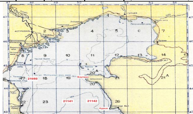
Схема расположения квадратов в средней части Каспийского моря
